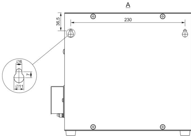
Габаритные и установочные размеры стабилизаторов напряжения переменного тока LIDER PS2000W-50
